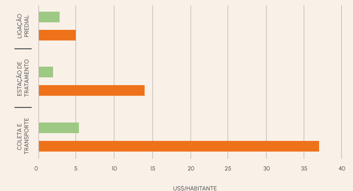
Gráfico 3: Composição de custos de sistemas centralizados e descentralizados em Dakar, Senegal (adaptado de Dodane, Sow, e Strande, 2012)
