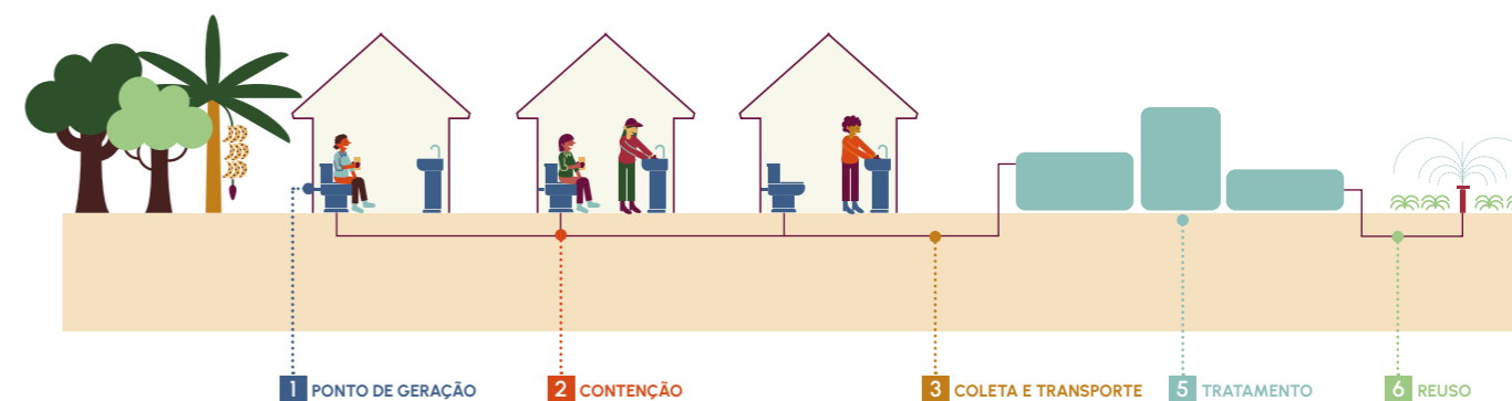
Figura 4: Possível arranjo das etapas em sistema centralizado
