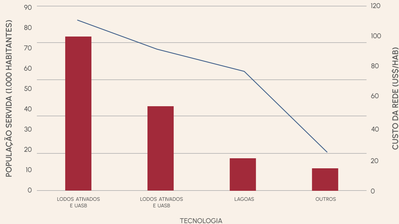
Gráfico 2: Custos médios de implementação e população média servida para ETEs de diferentes tecnologias financiadas pelo PRODES - ANA
